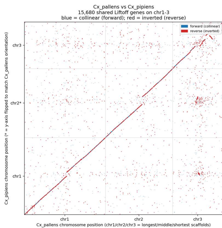
(D) pallens vs pipiens
